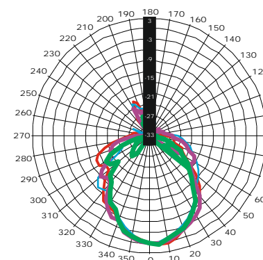
VERTICAL POLAR DIAGRAM — 4000 — 5000 — 6300 — 8000
