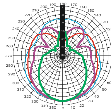
VERTICAL POLAR DIAGRAM — 250 — 500 — 1000 — 2000
